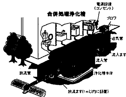
合併浄化槽のシステム
