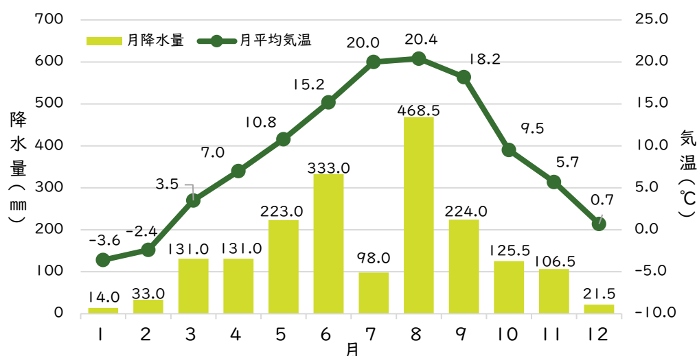
図3-6 気象庁の令和5(2023)年度における奥日光(日光)観測所の月降水量と月平均気温
