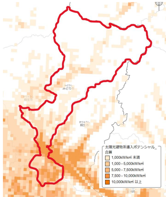
再生可能エネルギー情報提供システム【REPOS(リーボス)】から取得したコンテンツを加工して作成 図3-24 太陽光発電導入ポテンシャル(建物系の合計)
