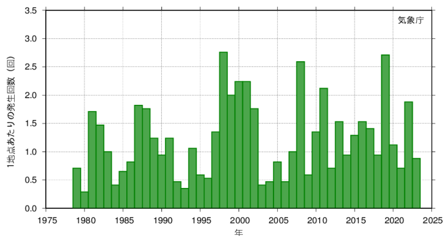
図3-11 群馬県の1時間降水量30mm以上の発生回数の推移
