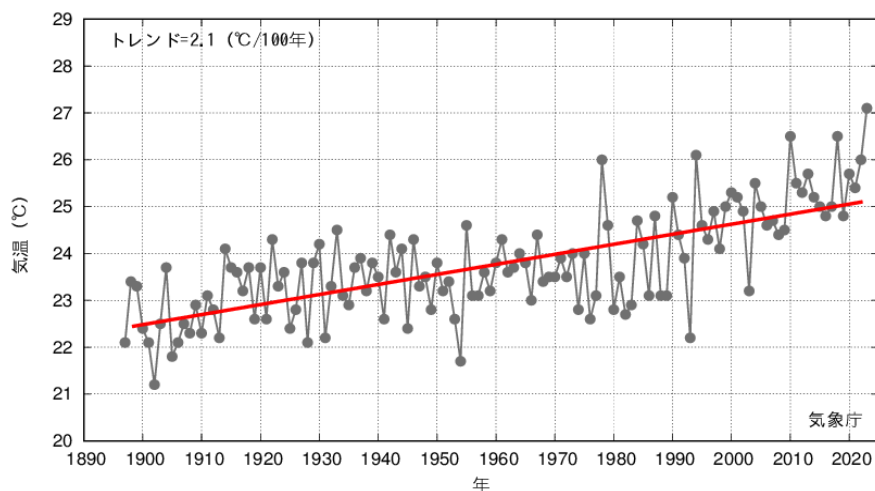
図3-7 前橋観測所における年平均気温の推移
