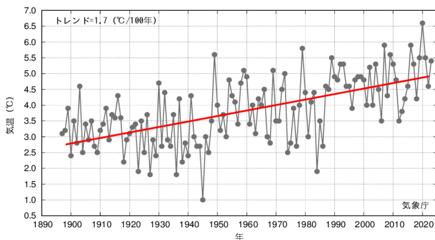
図3-8 前橋観測所における夏平均気温の推移
