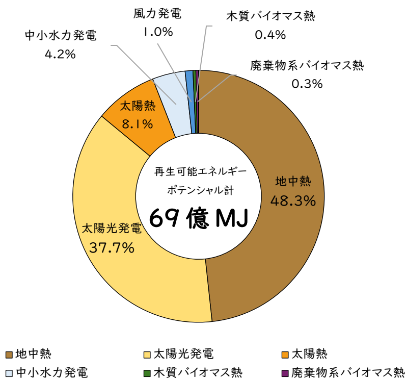
図3-31 再生可能エネルギー種別ポテンシャル
