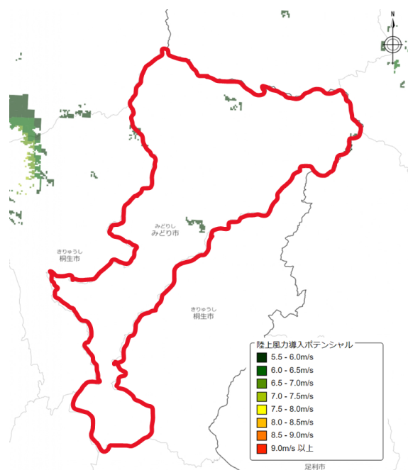
図3-26 陸上風力導入ポテンシャル
