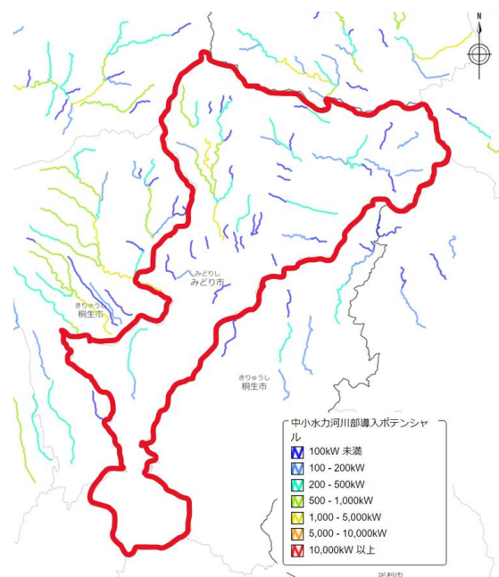
図3-27 中小水力発電導入ポテンシャル
