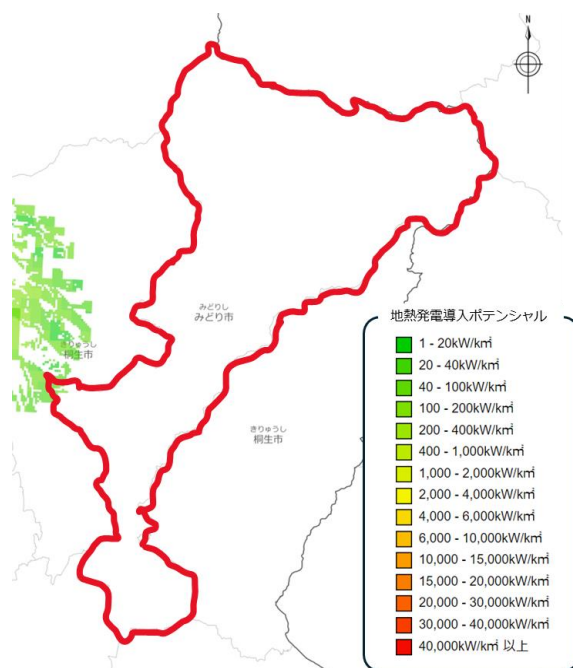
再生可能エネルギー情報提供システム【REPOS(リーポス)】から取得したコンテンツを加工して作成 図3-28 地熱発電導入ポテンシャル
