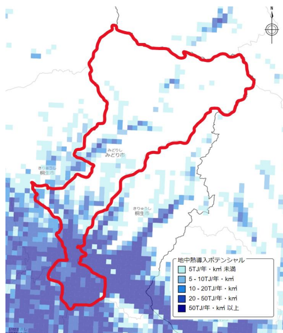
図 3-30 地中熱導入ポテンシャル
