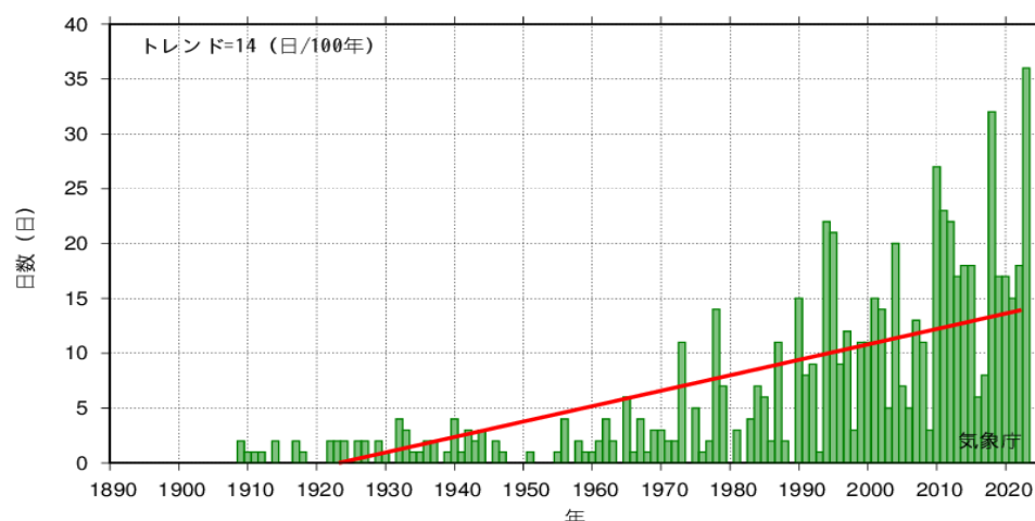
図3-10 前橋観測所における年間猛暑日日数の推移
