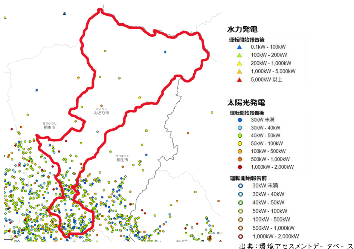
図3-23 FIT 認定設備の概略位置
