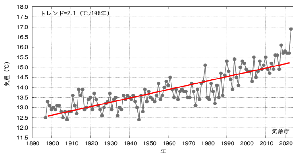
図3-7 前橋観測所における年平均気温の推移
