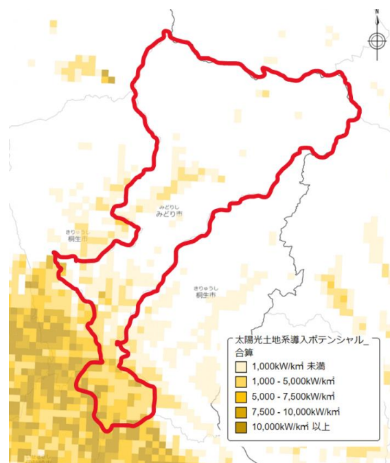
再生可能エネルギー情報提供システム【REPOS(リーボス)】から取得したコンテンツを加工して作成 図3-25 太陽光発電導入ポテンシャル(土地系の合計)
