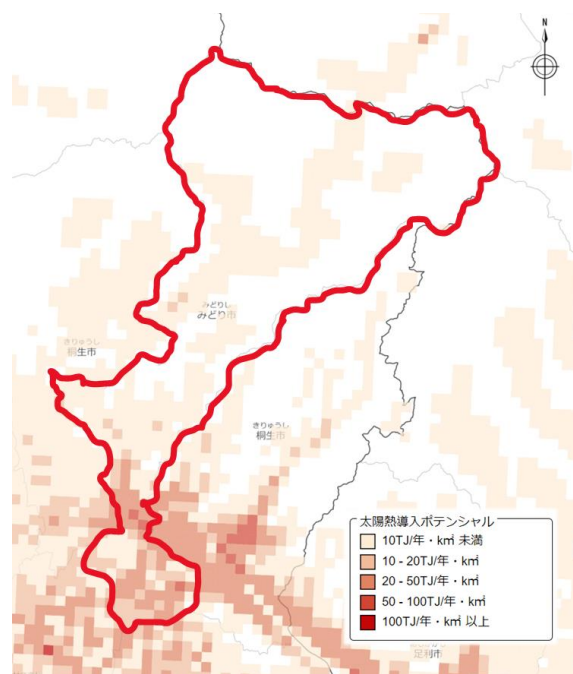
図 3-29 太陽熱導入ポテンシャル
